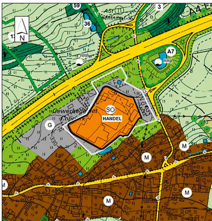
Flächennutzungsplan Planausschnitt
